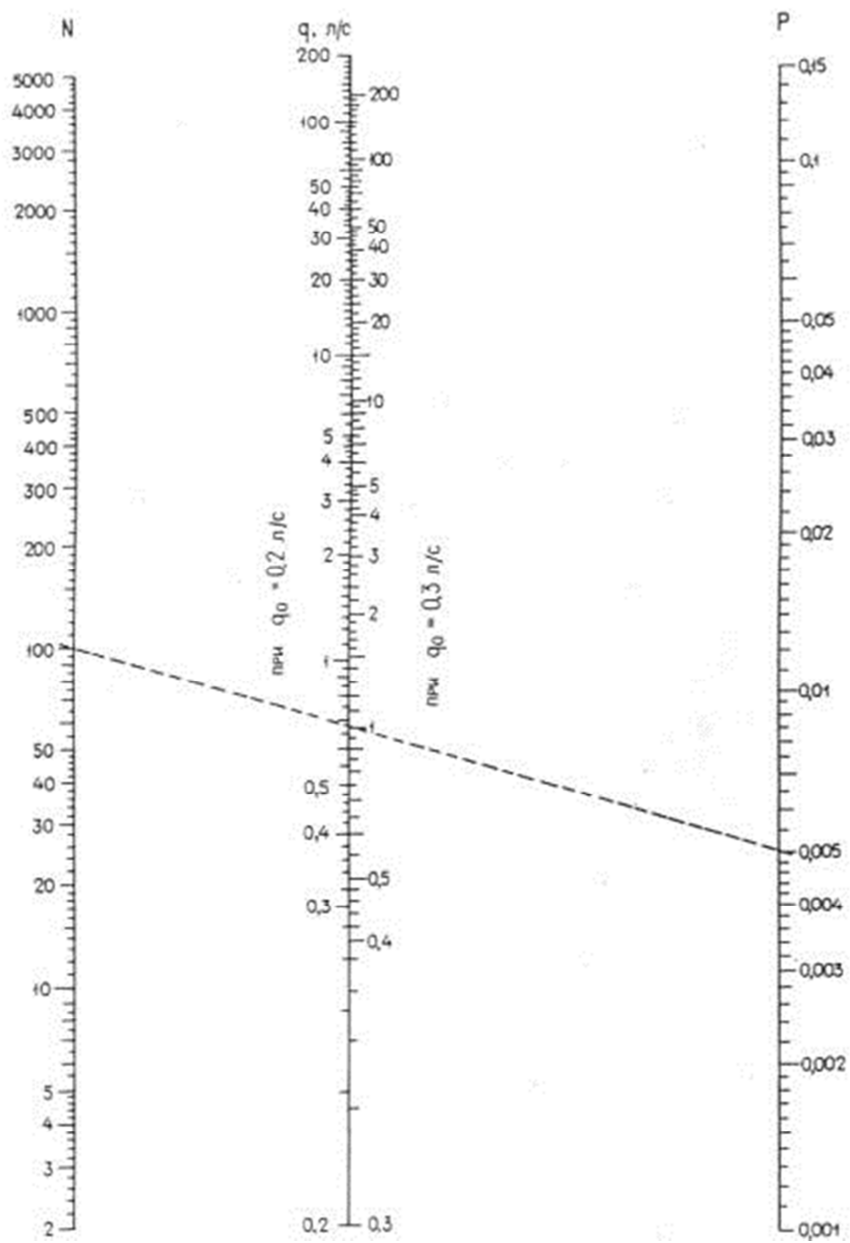
Черт. 2. Номограмма для определения секундных расходов
