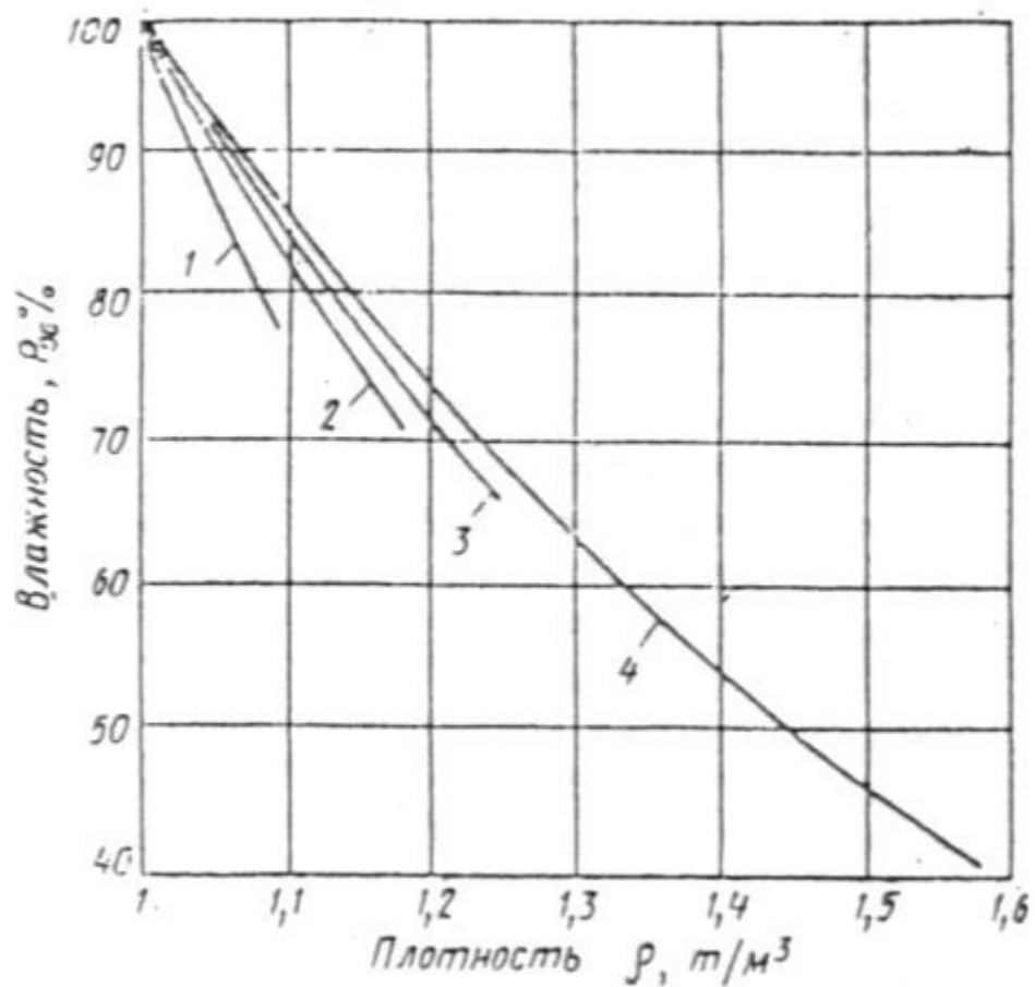
Рис. 5. Значения плотности в зависимости от влажности осадка станций осветления и обезцвечивания воды
