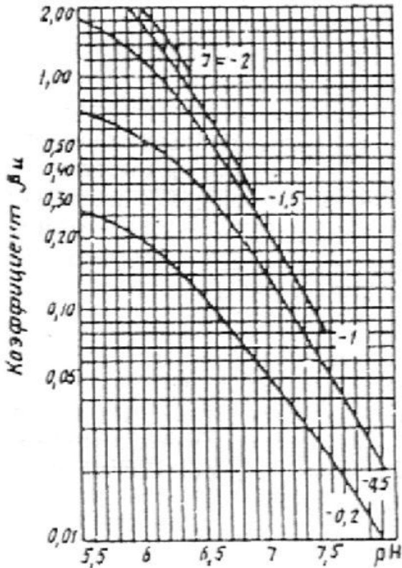
Рис. 4. Номограмма для определения коэффициента
