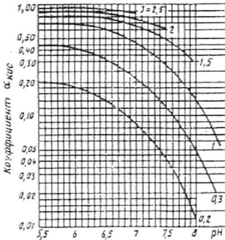
Рис. 3. Номограмма для определения коэффициента \alpha_{K_2CO_3}
