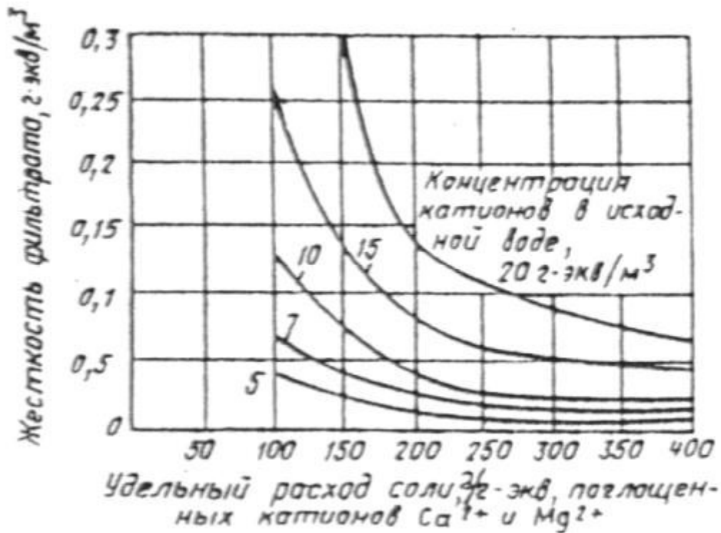
Рис. 1. График для определения остаточной жесткости воды, умягченной одноступенчатым натрий-катионированием
