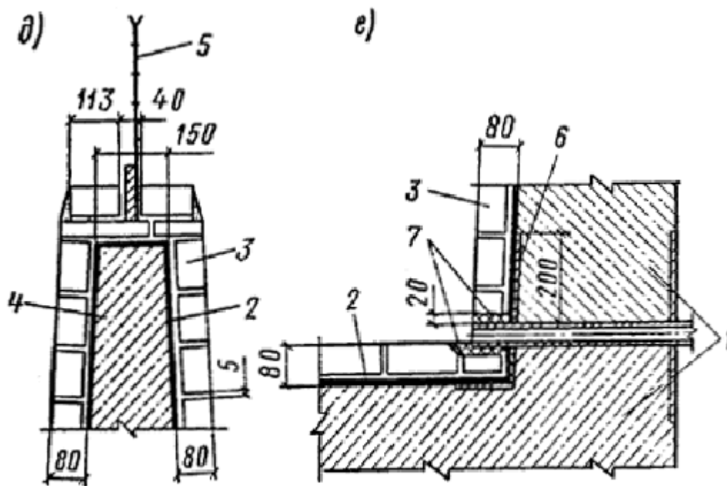
Рис. 1. Емкость для хранения сернокислого алюминия (перекрытие — съемные деревянные щиты)
