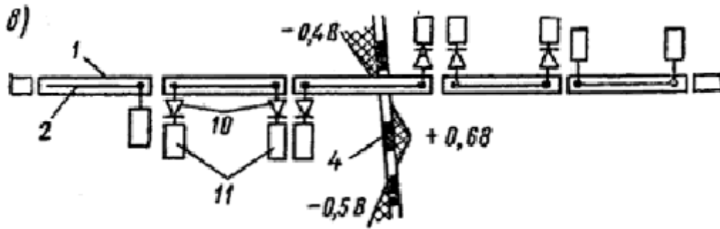
Рис. 1. Схемы защиты блочной железобетонной конструкции
