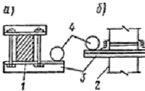
Рис. 1. Примеры выполнения держателей из электроизоляционных материалов для крепления трубопроводов
