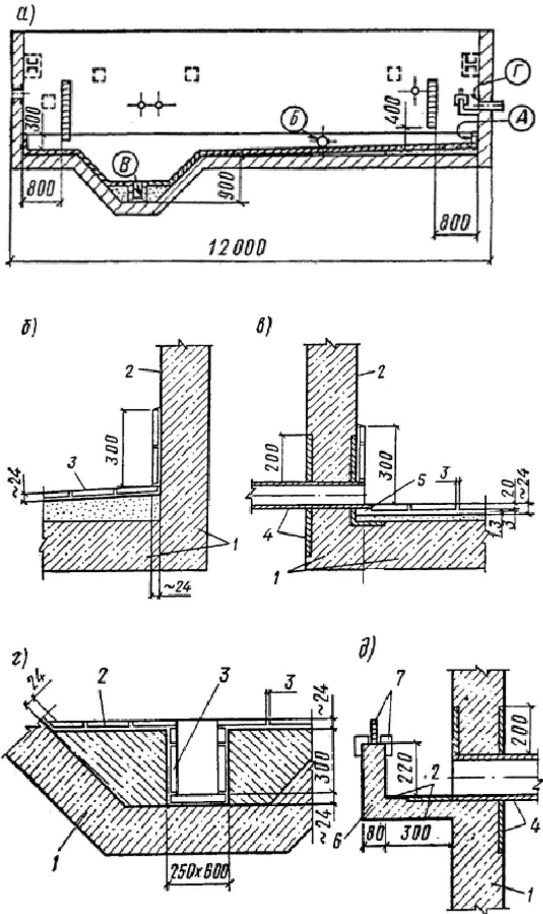
Рис. 3. Нефтеловушка (перекрытие — съемные деревянные щиты)
