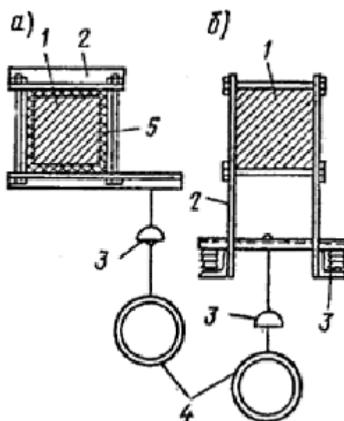
Рис. 2. Примеры выполнения металлических держателей для крепления трубопроводов
